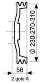
Puleggia Pulley Polea Poulie Keilriemenscheibe
